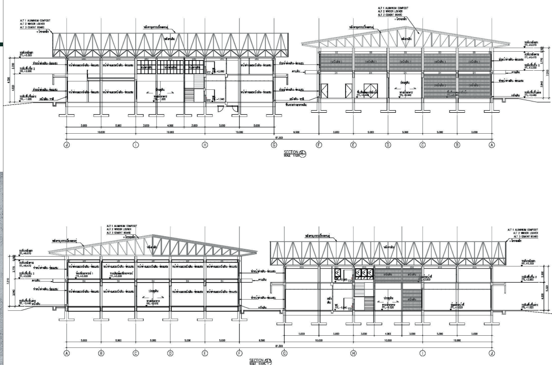
แบบเต็มของ อาคาร ประลองวิศวกรรมโครงสร้าง และ วิศวกรรมชลศาสตร์ และลักษณะการใช้งานในปัจจุบัน
